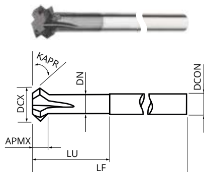
DCX ≥ 8 mm Spitze abgeflacht
