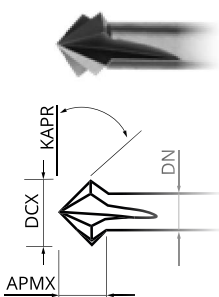
DCX ≤ 6 mm Stirn spitz zulaufend
